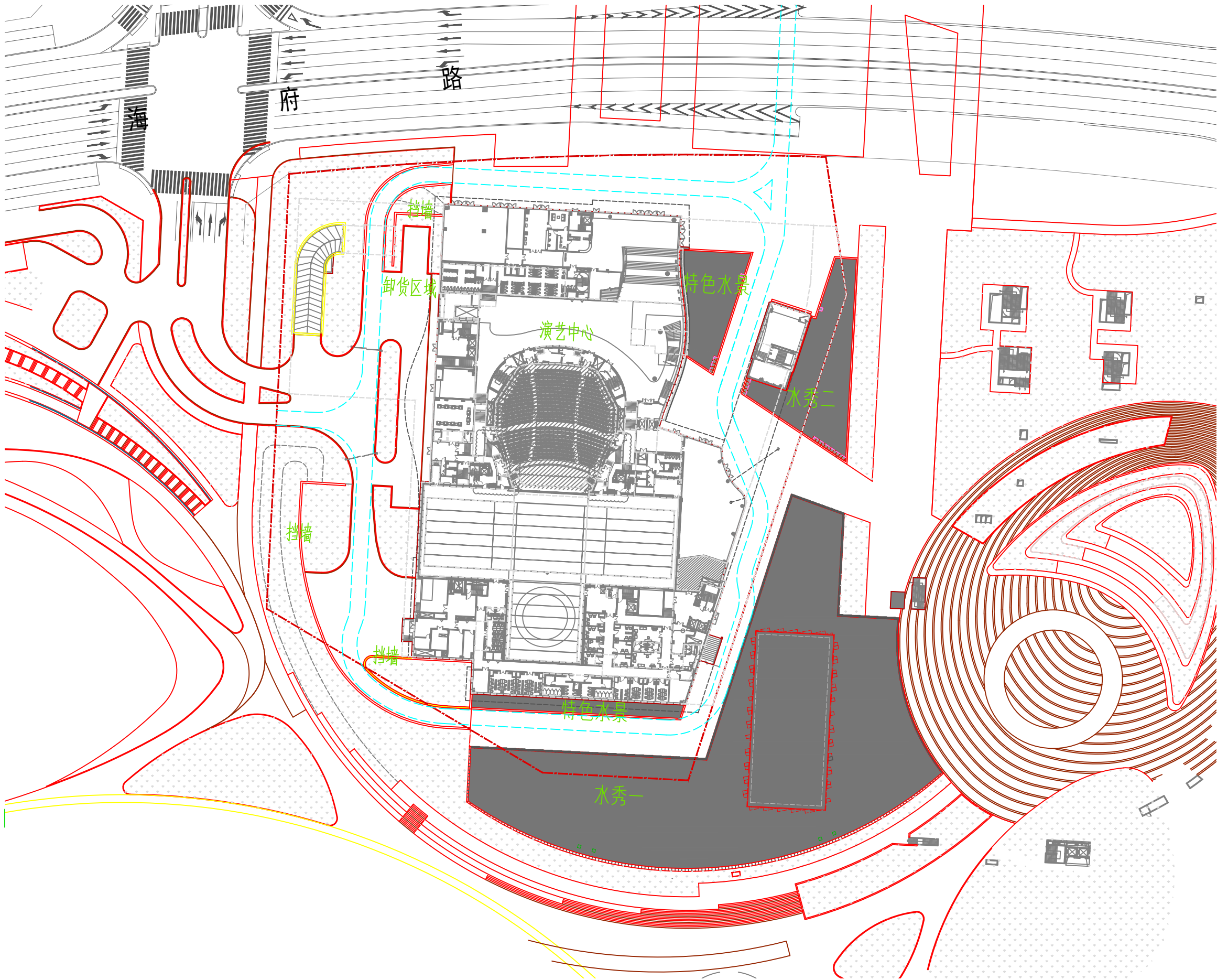
① 总平面布置图 1: 500
